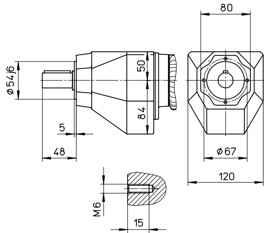
B14 Вариант с фланцевым монтажом лапы
