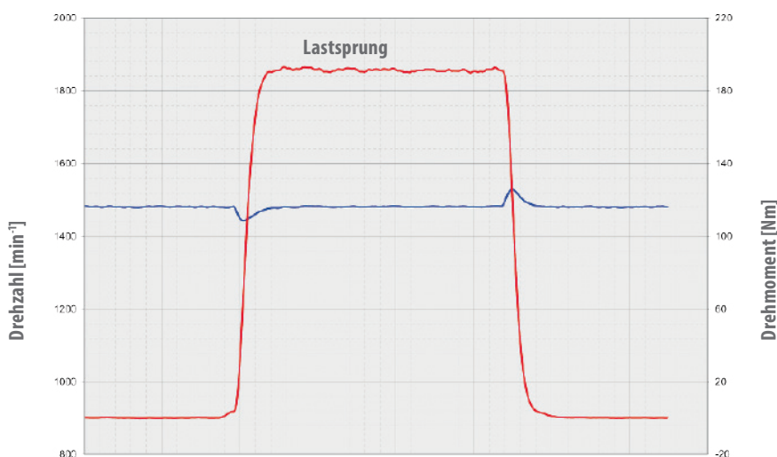
Dynamisches Ausregelverhalten einer Last
