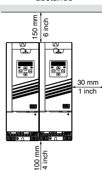
Einbaulage und Mindestabstände
