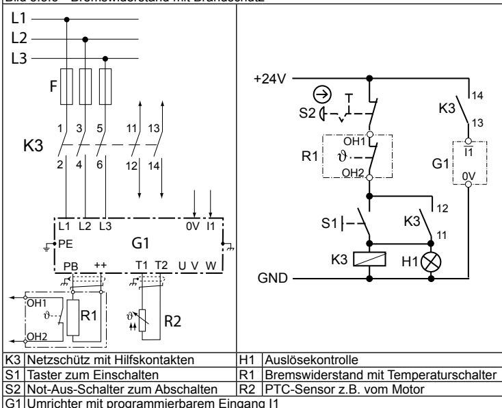
Bild 3.3.6 Bremswiderstand mit Brandschutz
