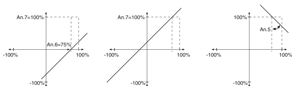
Fig. 6.2.7.c X-Offset (An.6)=75%; Y-Offset (An.7)= 100%; amplification. (An.5)= -1.00
