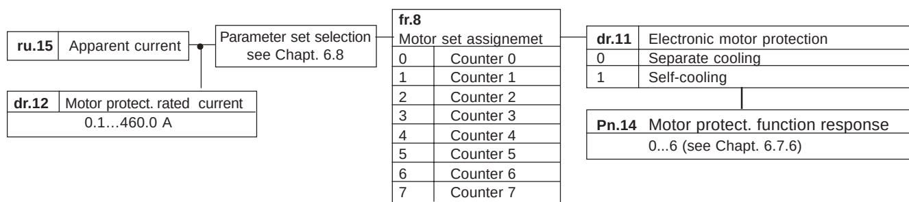
Fig. 6.7.8.a Motor protection mode
