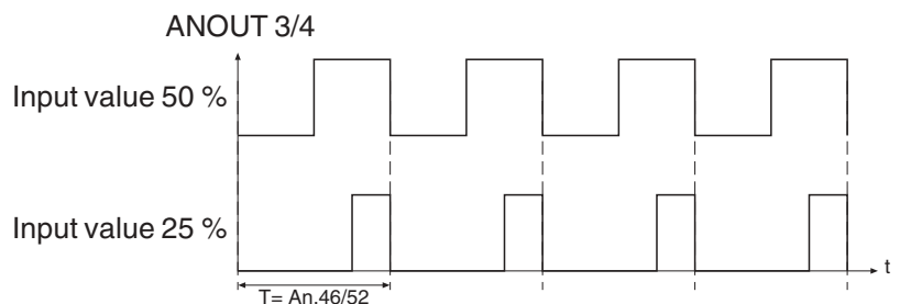
Bild 6.2.11.a PWM - output signal
