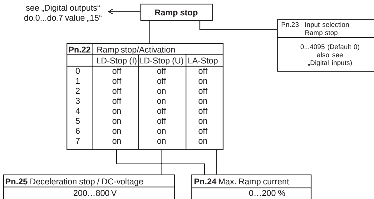
Fig. 6.7.1.a Survey ramp stop function
