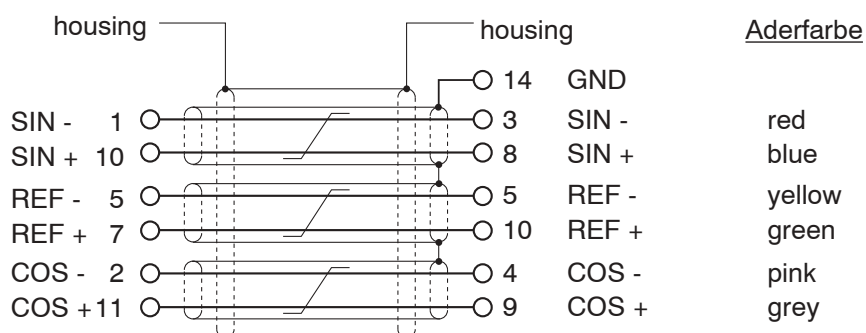
Bild 6.10.2.c Resolver cable
