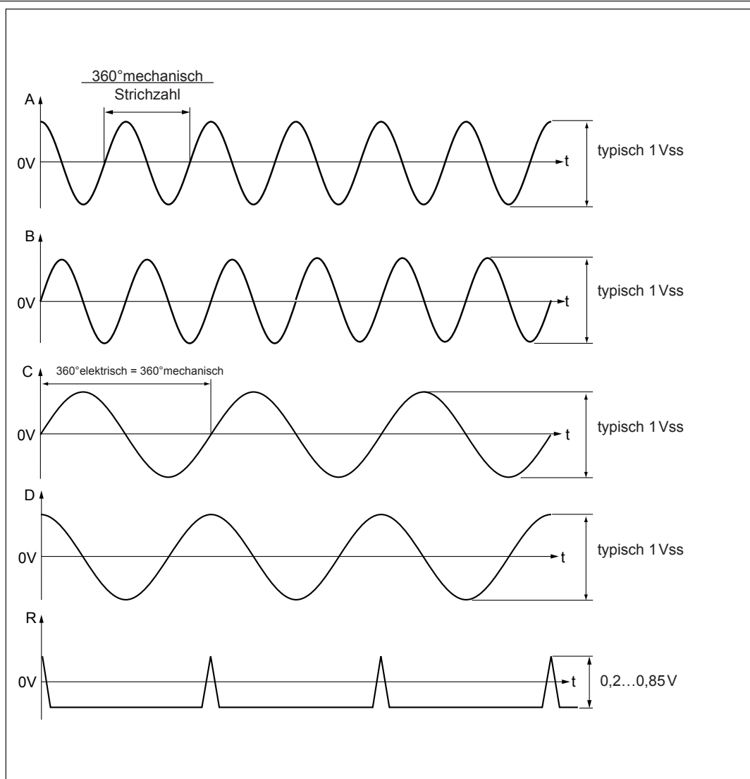
Bild 3.2.3.1 Signalspuren
