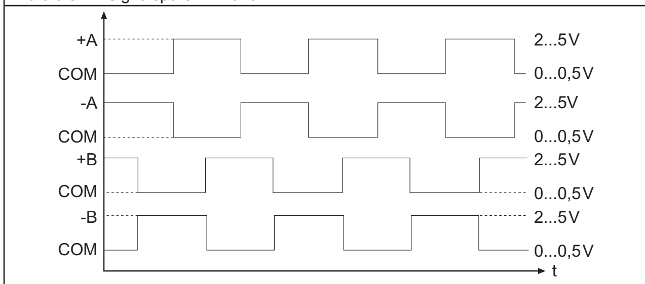
Bild 3.3.3.1 Signalspuren A+ und B+
