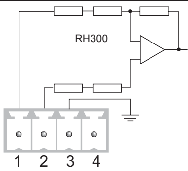
Stecker X3B und Innenschaltung
